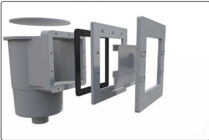
Explosionsdarstellung Skimmer
