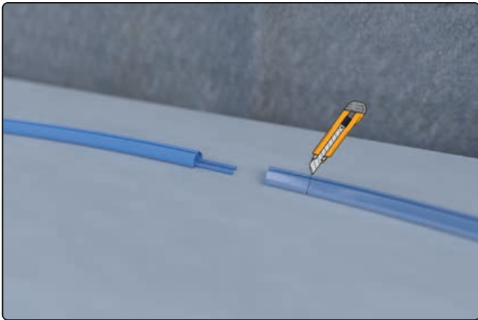
Spaltmaß >1cm / Bodenschiene kürzen
