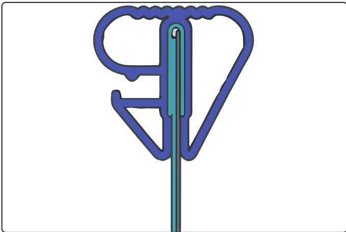
Querschnitt Handlauf mit Einhängebiese
