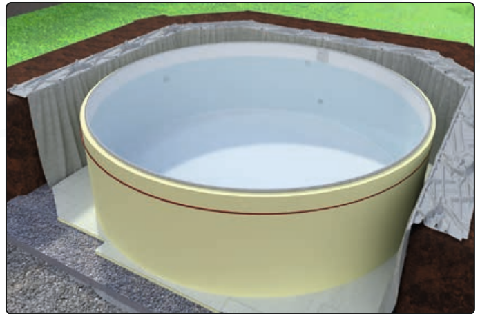
Die Rundschalungselemente sollten mit einem Gurt oder einem ähnlichen Befestigungsmittel fixiert werden.
