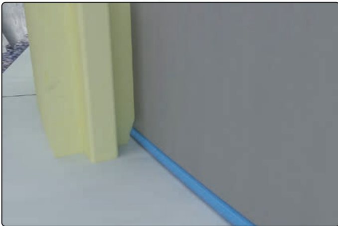
Die Rundschalung sollte an der Bodenschiene um 45° angeschrägt werden
