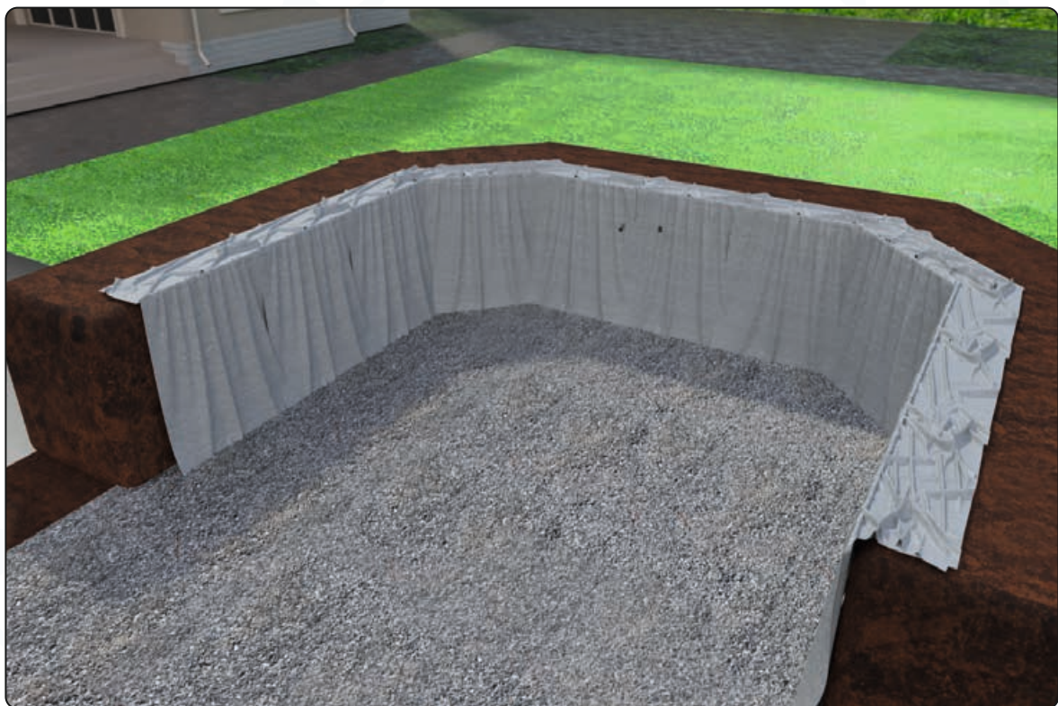
Falls erforderlich: Baugrube mit zusätzlicher Schotter- und Geotextilschicht ausgekleidet
