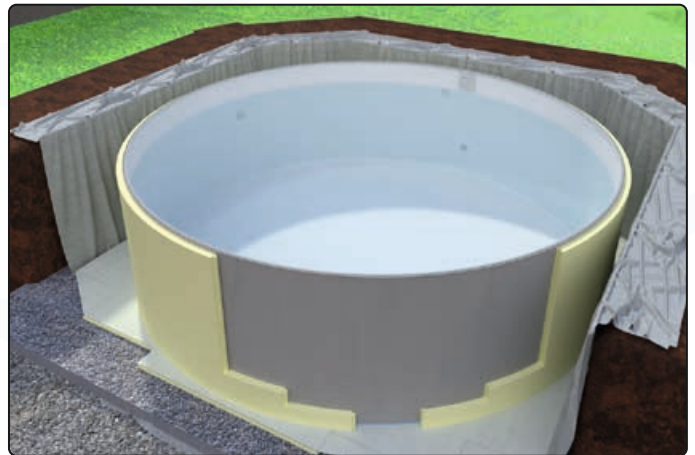
Rundschalung zusammenstecken. 15cm Elemente unten
