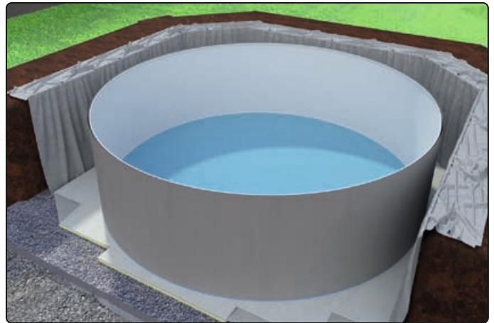
Füllen Sie etwa 3 mm Wasser in den Pool und glätten Sie die Bodenfalt
