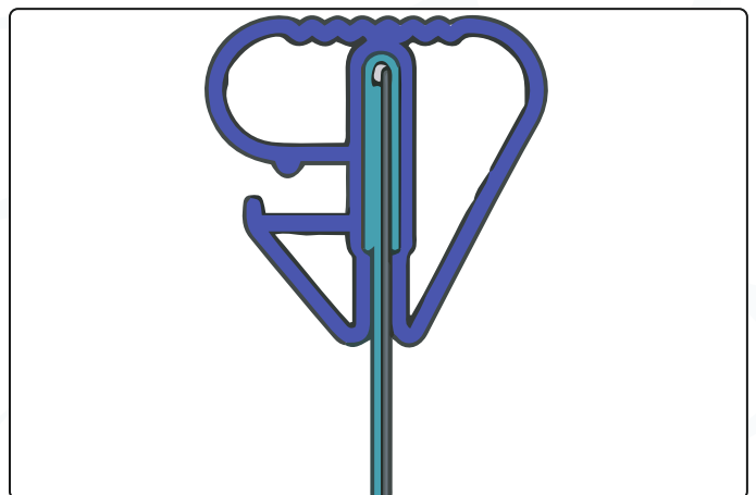
Querschnitt Handlauf mit Einhängebiese
