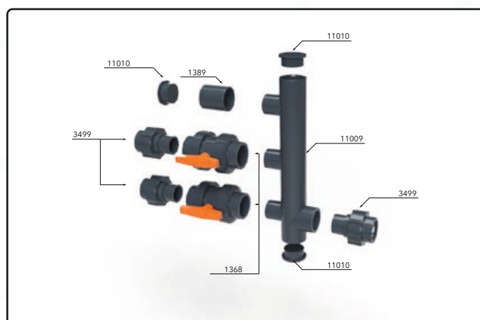
Anschluss Zirkulationsverteiler
