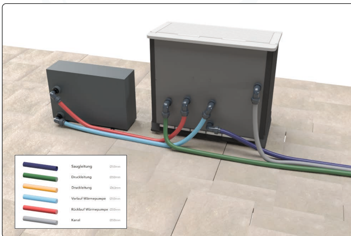
Technikbox Rückseite (Verrohrung ohne optionaler Saugdüse ) !! Achten Sie auf die Beschriftung der Abgänge in der Technikbox !!
