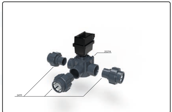
Anschluss PVC- U 3 Wege Drehscheibenventil
