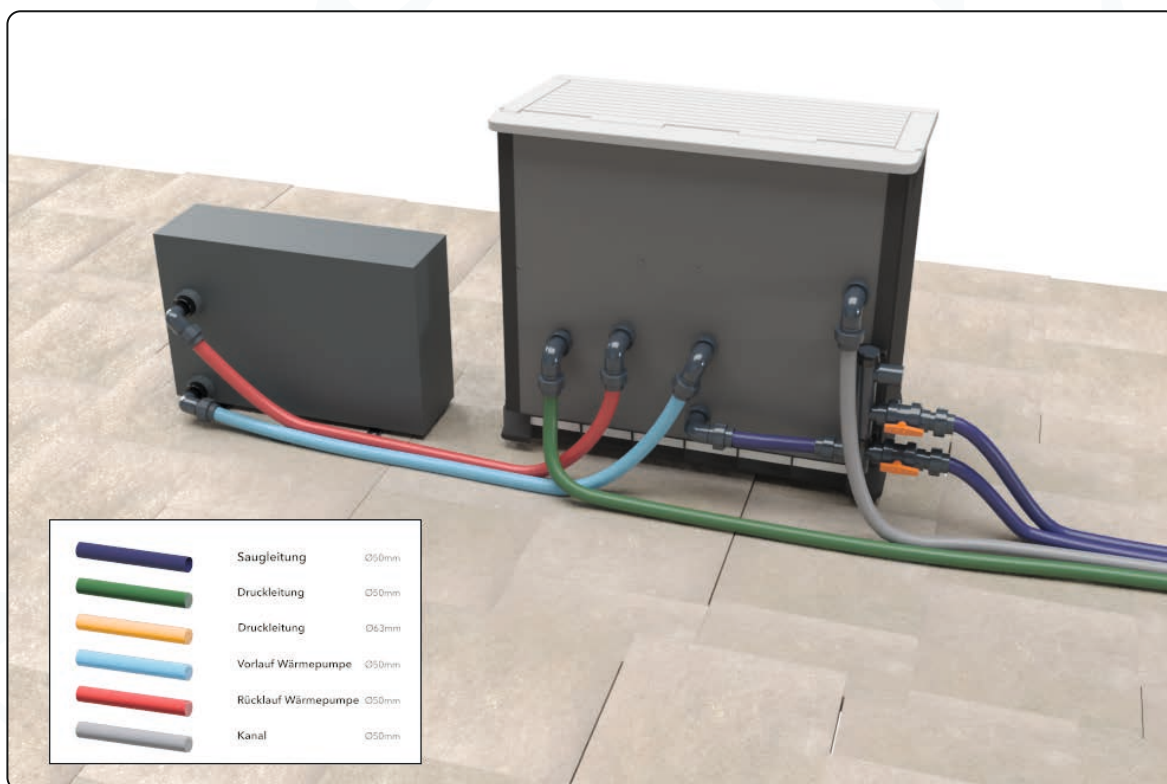
Technikbox Rückseite (Verrohrung mit optionaler Saugdüse ) !! Achten Sie auf die Beschriftung der Abgänge in der Technikbox !!
